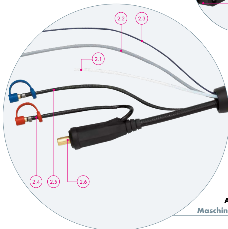
Abbildung 1: Brenner-Schnittstelle
