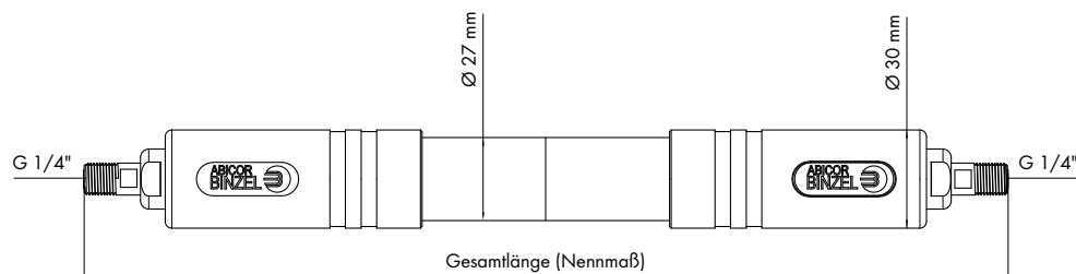
Längendarstellung
