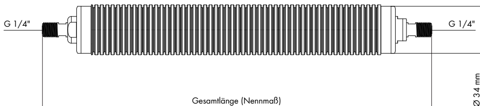
Längendarstellung
