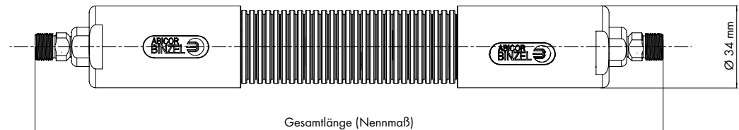
Längendarstellung
